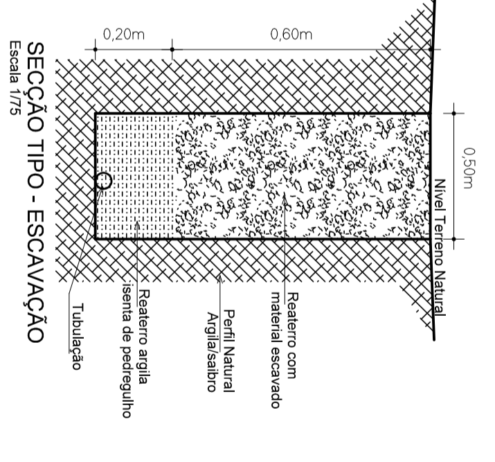
DETALHE RESERVATÓRIO
